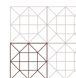
GOZZANO 400X400 SP. MM 15-22 Prelevigato Spazzolato Piallato a mano Sabbiato
